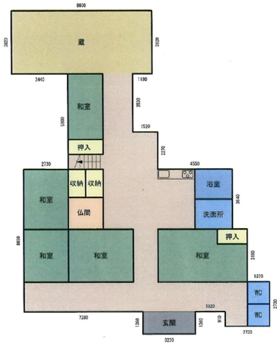
平面詳細図（1階）
